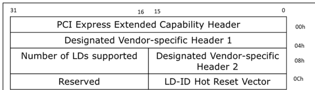
Figure 8-7. MLD DVSEC
